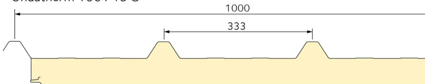
Ondatherm 1001 TS G
